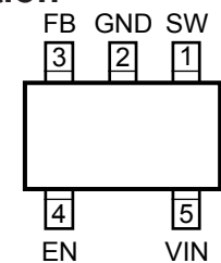
TSOT-23-5 (BD5)
