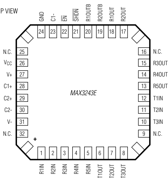
TQFN-EP
