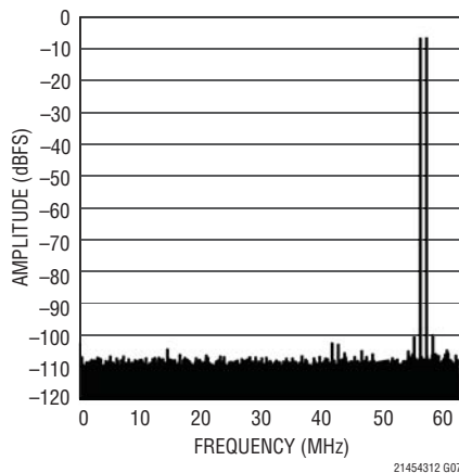
FFT, f_{IN} = 69\text{MHz} , 70\text{MHz} , -7\text{dBFS} , 125Msps
