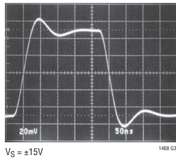
Small-Signal Transient, AV = -1
