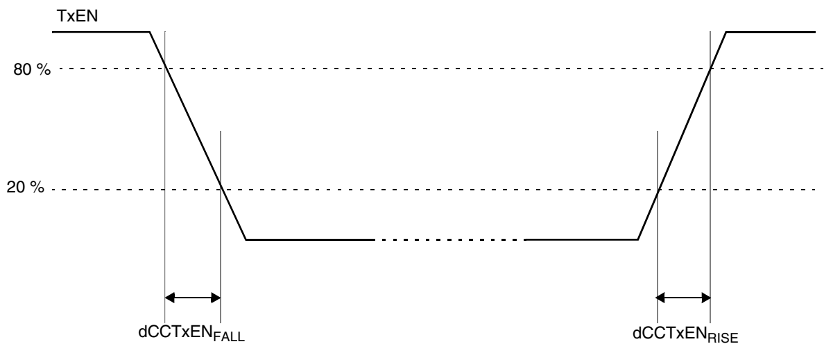
Figure 31. TxEN signal
