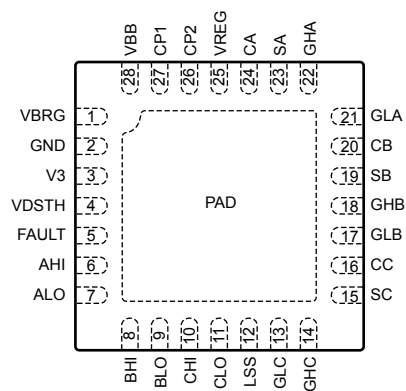
A4919GETx-3 variant
