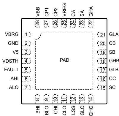
A4919GETx-5 variant
