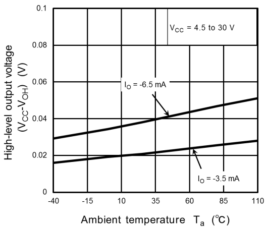
Fig. 13.2.6 (V_{CC}-V_{OH}) - T_a
