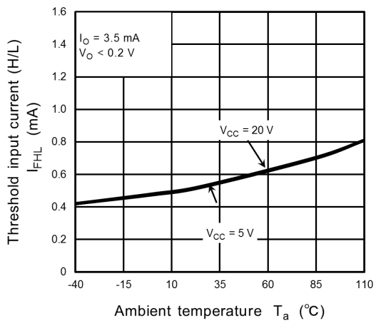
Fig. 13.2.2 I_{FHL} - T_a
