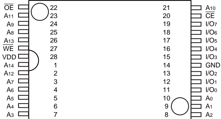
(FPT-28P-M19)
