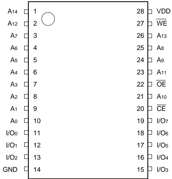
(FPT-28P-M17 / FPT-28P-M01)
