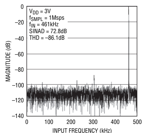
461kHz Sine Wave 8192 FFT Plot
