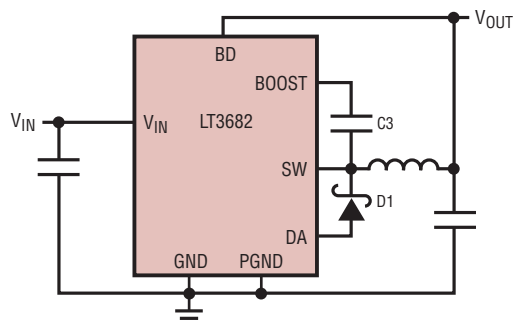
(5a) For V_{\text{OUT}} > 2.8\text{V} ; V_{\text{IN(MIN)}} = 4.3\text{V} if V_{\text{OUT}} < 3\text{V}
