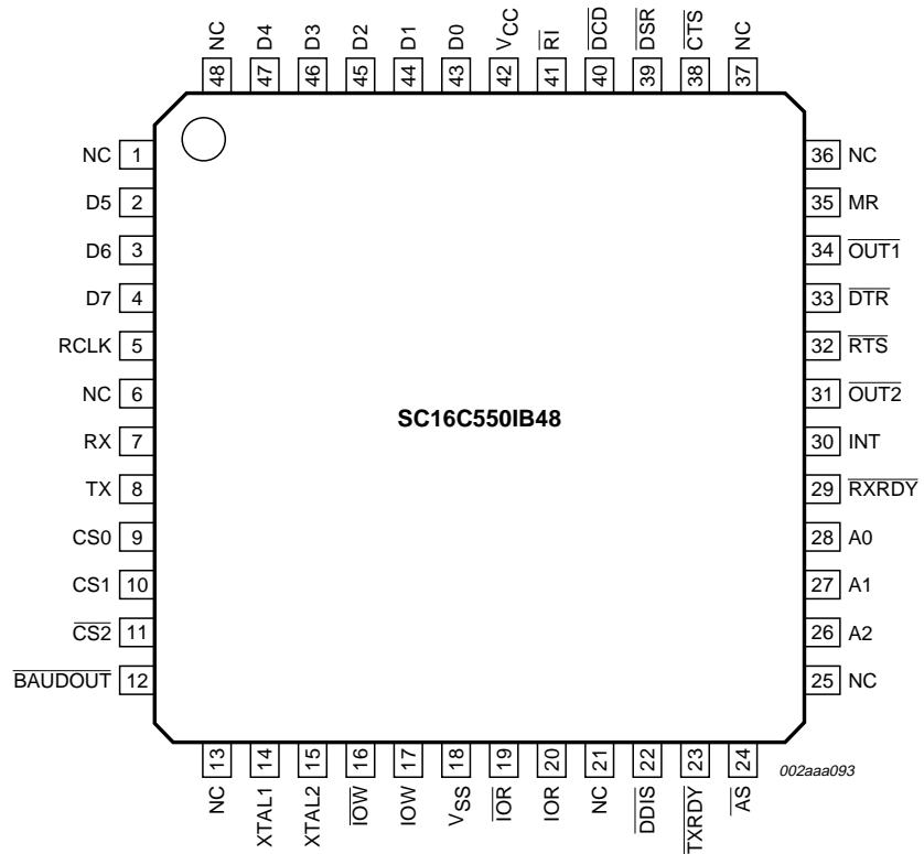
Fig 3. LQFP48.
