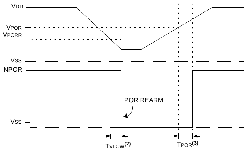
FIGURE 23-1: POR AND POR REARM WITH SLOW RISING V_{DD}
