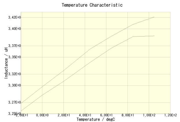
NLCV32T-3R3M-PF(DC = 0A)
