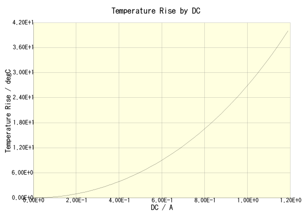
NLCV32T-3R3M-PF(Amb. Temp. = 20degc)
