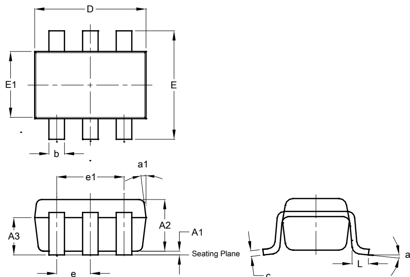
SOT26 (SC74R)
