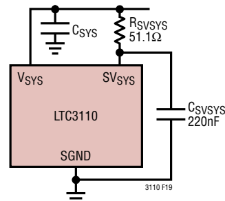
Figure 16. SV_{SYS} Filtering
