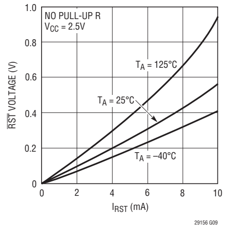
RST V_OL vs I_RST
