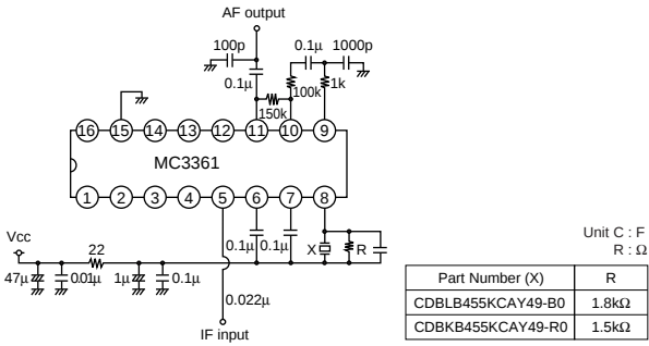
MC3361
