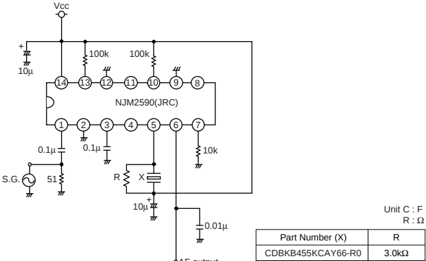
NJM2590
