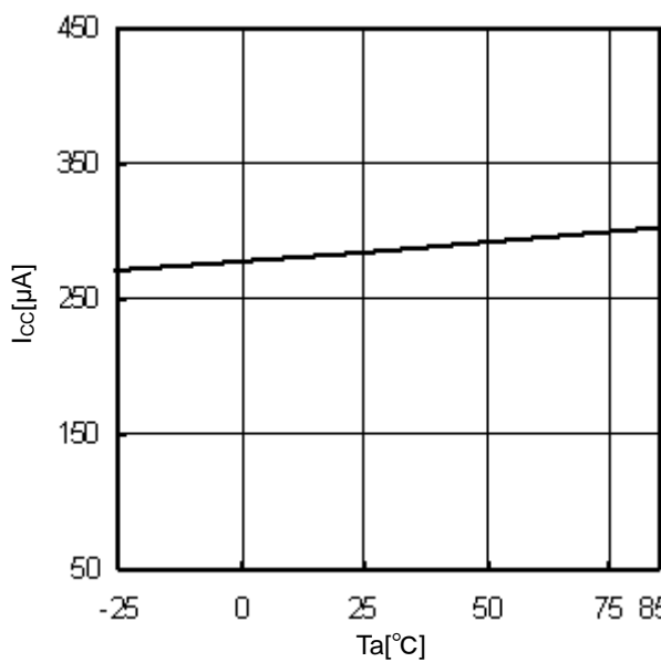
Fig.10 Ta- I_{CC}
