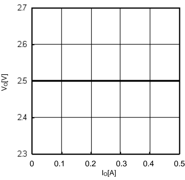
Fig.13 I_O - V_O
