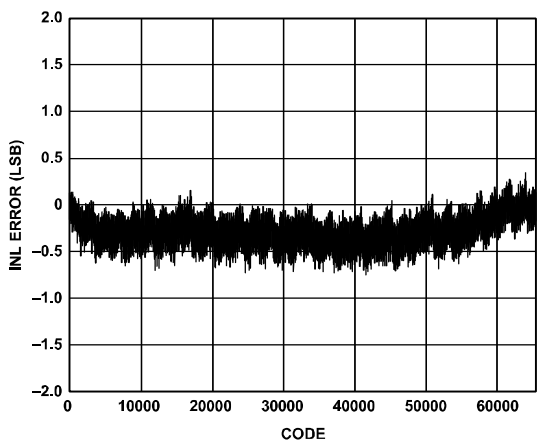
图15. 典型INL误差, \pm 5 V范围
