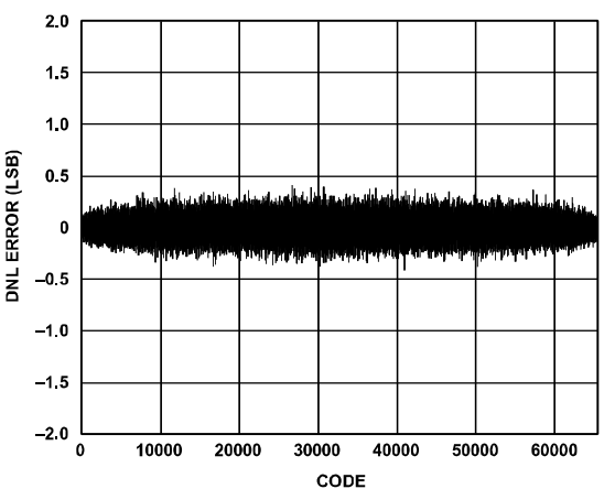
图16. 典型DNL误差, \pm 10 V范围
