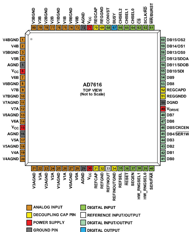
图7. 引脚配置
