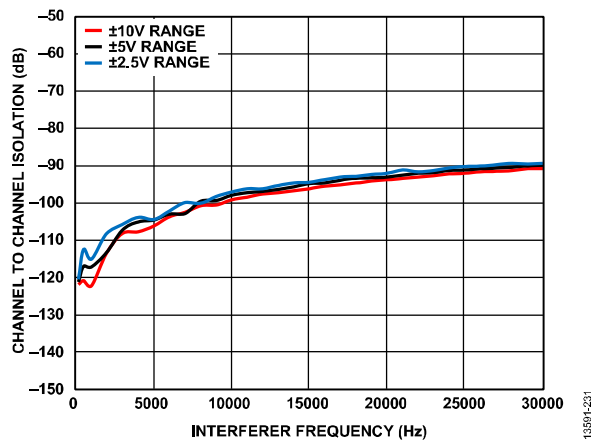
图31. 通道间隔离
