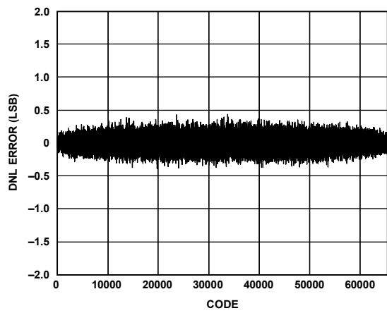
图17. 典型DNL误差, \pm 5 V范围
