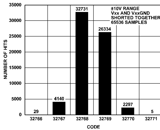
图18. 码中心处的码直流直方图, \pm 10 V范围
