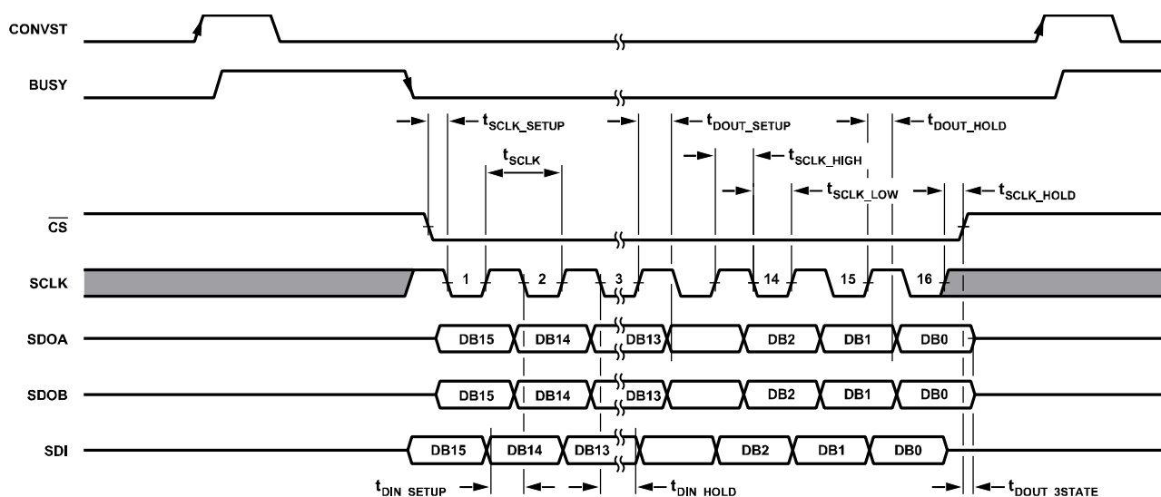
图6. 串行时序图
