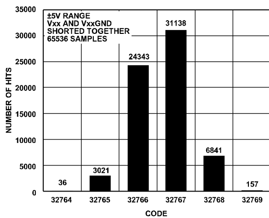
图19. 码中心处的码直流直方图, \pm 5 V范围
