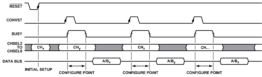
图51. 硬件模式通道转换设置
