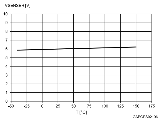
Figure 34: V_{senseh} vs. T_{case}
