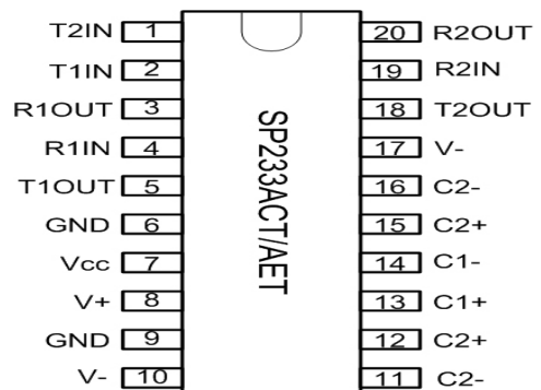
20 pin WSOIC
