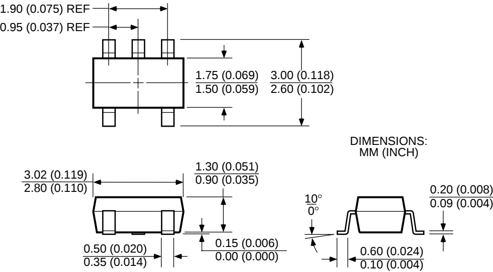
SOT-23-5 (M)
