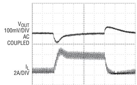
Load Step (Pulse Skip Mode)
