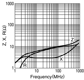
HF70ACC201209
