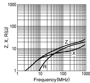
HF50ACC201209
