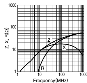
HF50ACC321611
