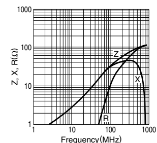
HF30ACC322513
