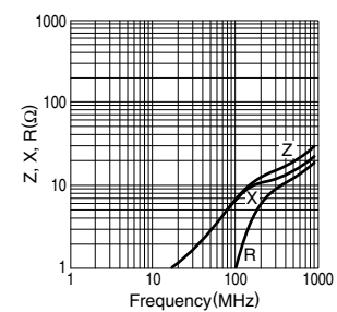
HF30ACC201209
