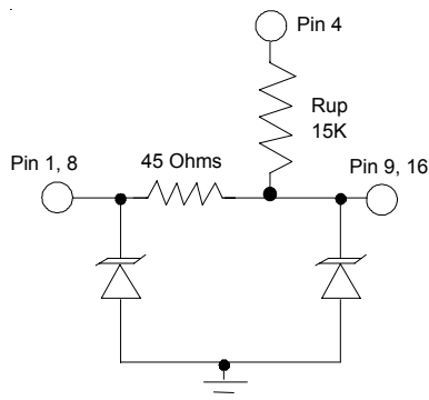
DAT1, DAT2
