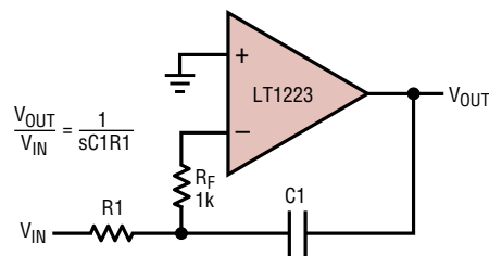
LT1223 • TA06
