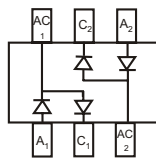
BAT54SDW*
