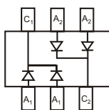
BAT54CDW*
