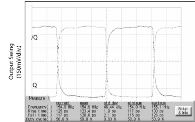
155MHz Output
