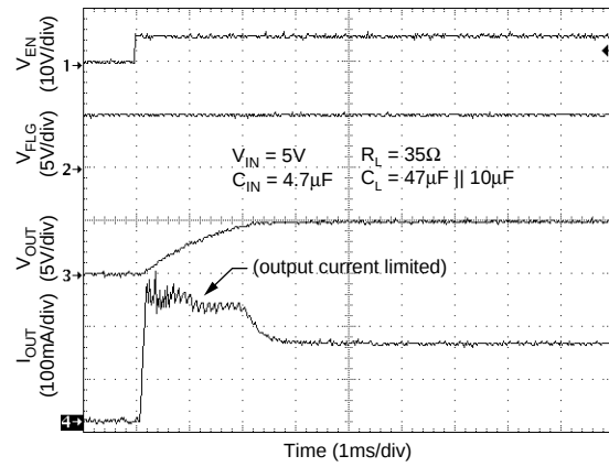
Turn-On (MIC2536-1)
