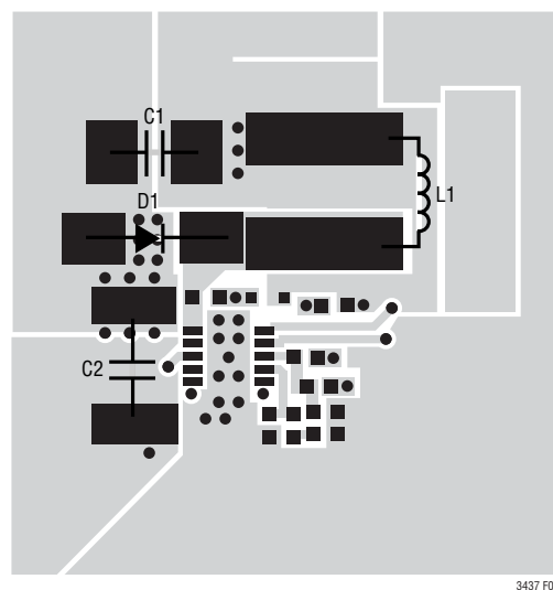
DD Package Topside Metal
