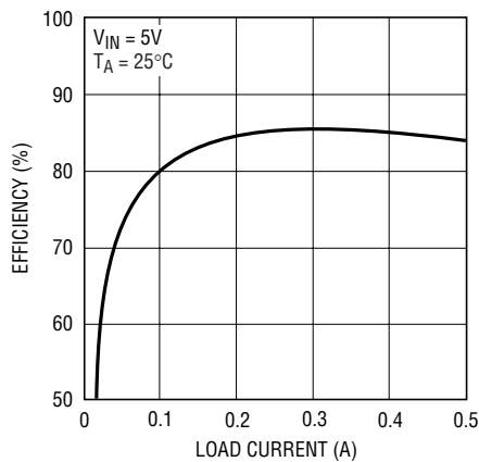
Efficiency, AV DD = 13V
