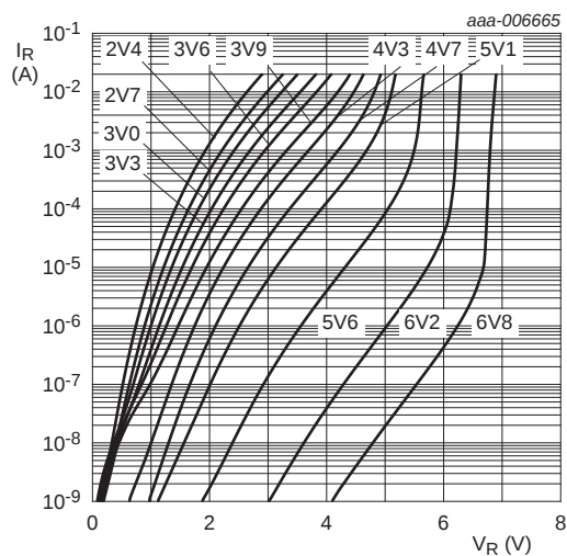
BZX84-A/B/C2V4 to BZX84-A/B/C6V8 T amb = 25 °C
