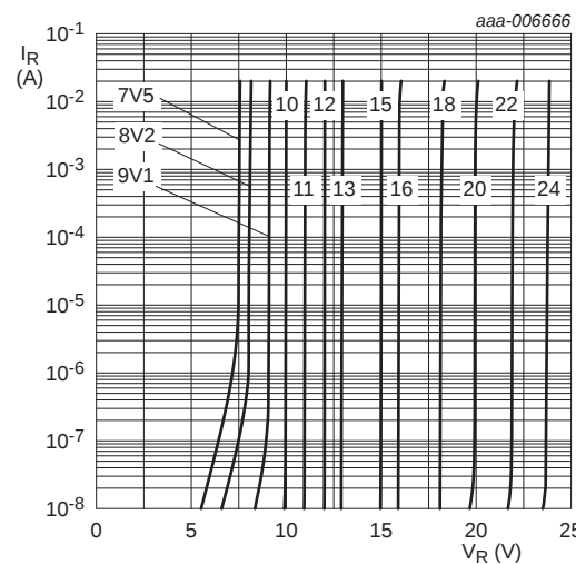
BZX84-A/B/C7V5 to BZX84-A/B/C24 T amb = 25 °C
