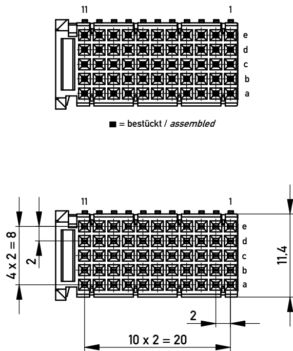
Bestückungsplan / contact layout
