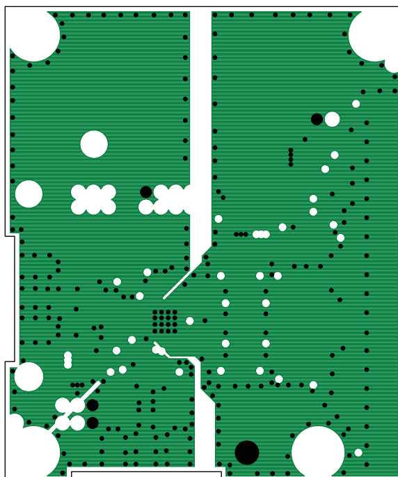
Inner Layer 2 GND
