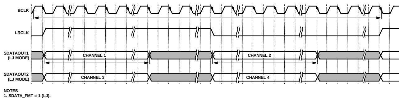
Figure 25. LJ Audio Format
