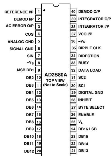
DIP (D) Package
