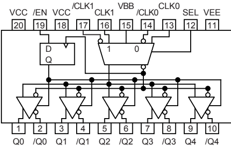
20-Pin TSSOP
