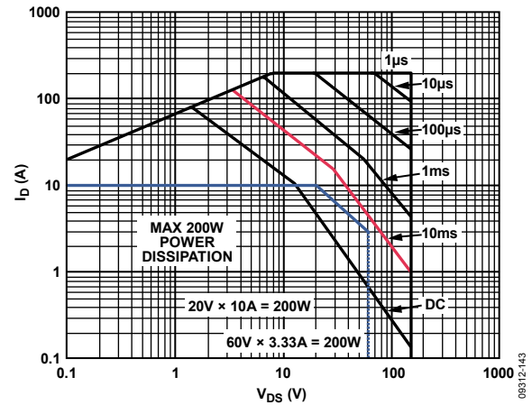
Figure 49. FET SOA
