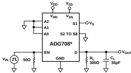
Figure 26. Enable Delay, t ON (EN), t OFF (EN)
