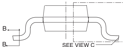
VIEW A-A
