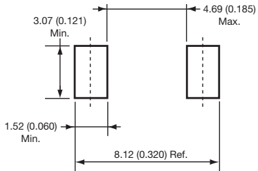
DO-214AB (SMC)
