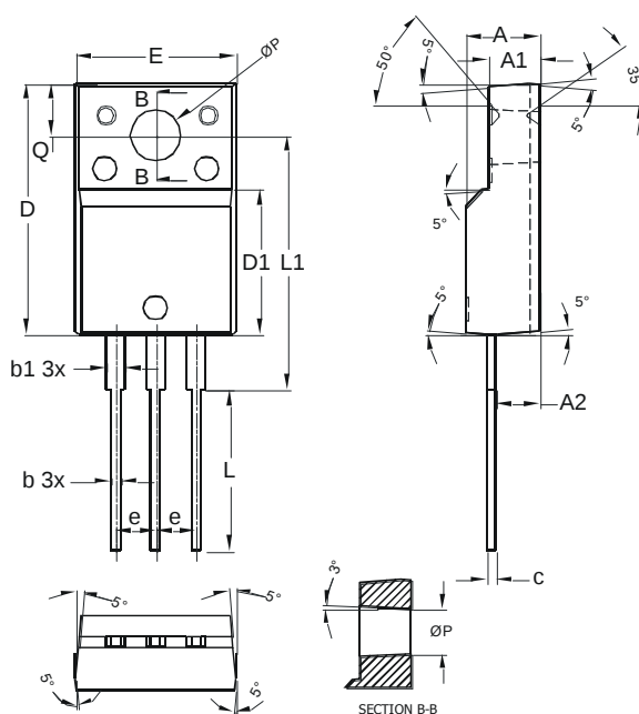
ITO220AB
