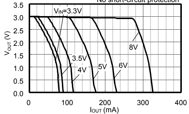
S-812C30A (Ta=25°C)
