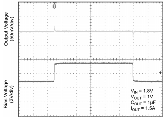
Line Transient ( V_{BIAS} )
