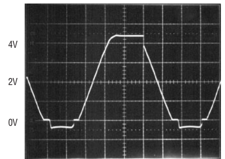
LT2078/LT2079 NO PHASE REVERSAL
