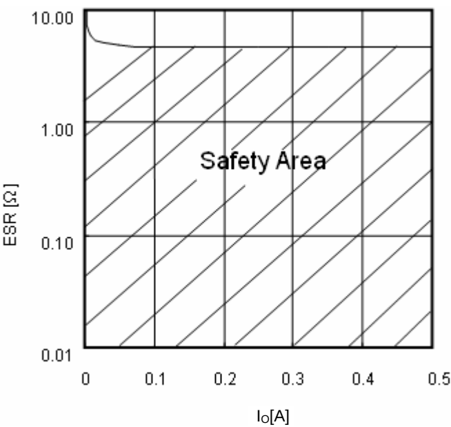
Fig.19 ESR condenser
