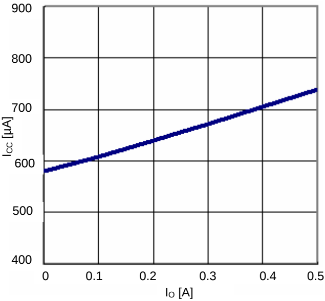
Fig.20 I_o - I_{cc}
