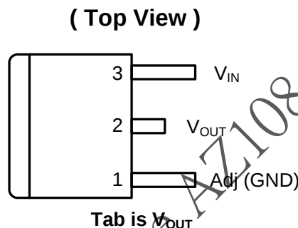
(2) TO263-3L
