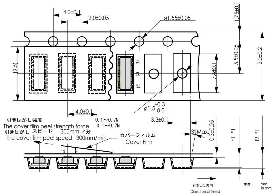
第3図 プラスチックテープの外形寸法図 Figure 3. Dimensions of Plastic Tape (CSTCC3M68G53A-R0)
