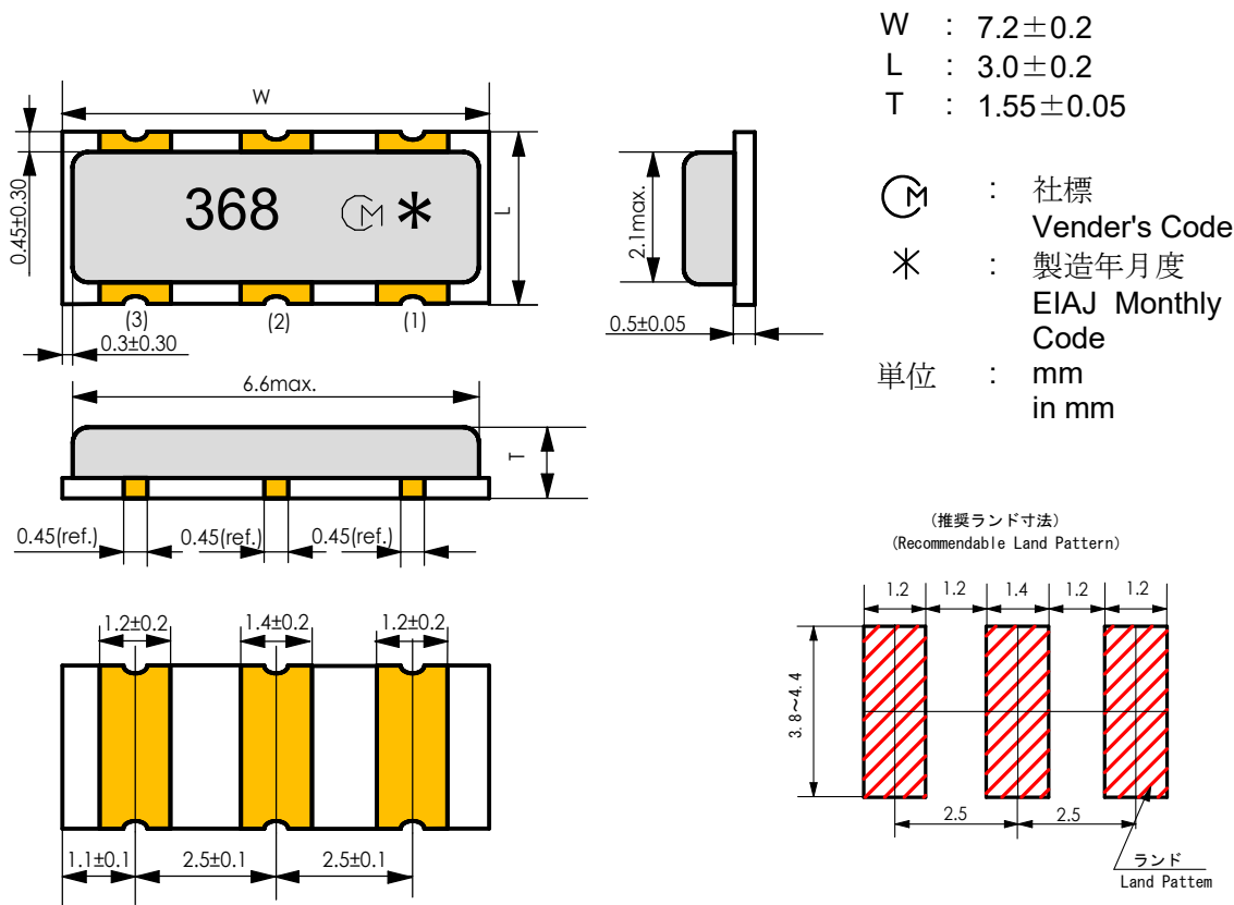
第1図 外形寸法図 Figure 1. Dimensions
