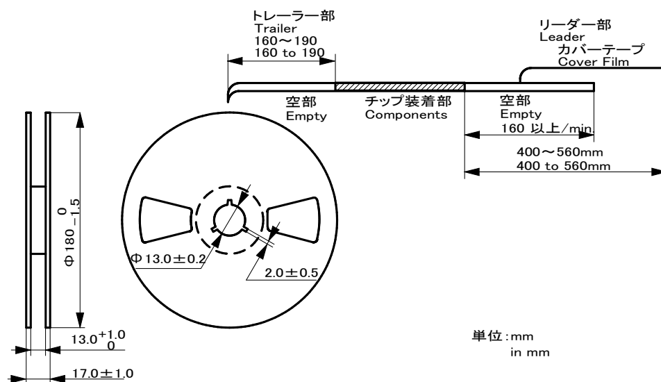
第4図 プラスチックリールの外形寸法図 Figure 4. Dimensions of Plastic Reel (CSTCC3M68G53A-R0)
