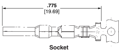
Socket
