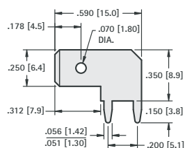
.250 (6.4) TAB
