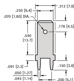
.250 (6.4) TAB
