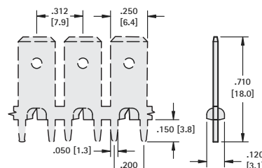
.250 (6.4) TAB
