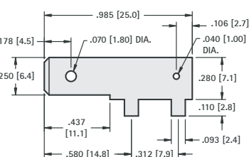
.250 (6.4) TAB
