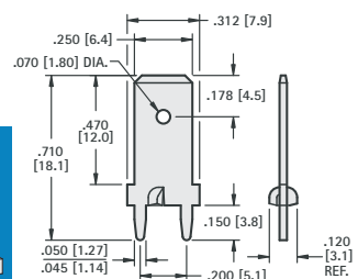
.250 (6.4) TAB
