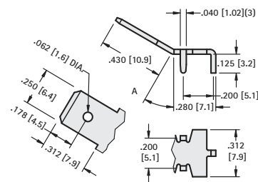
.250 (6.4) TAB
